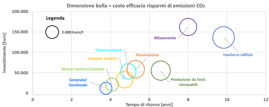
Figura 6.7 – Risparmi potenziali di emissioni di CO 2 : diagramma a bolle con costo efficace del risparmio di emissioni, investimento e tempo di ritorno.
