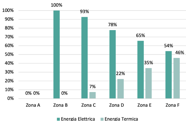
Figura 4.5 - Differenziazione percentuale consumi elettrici e termici nelle zone climatiche.
