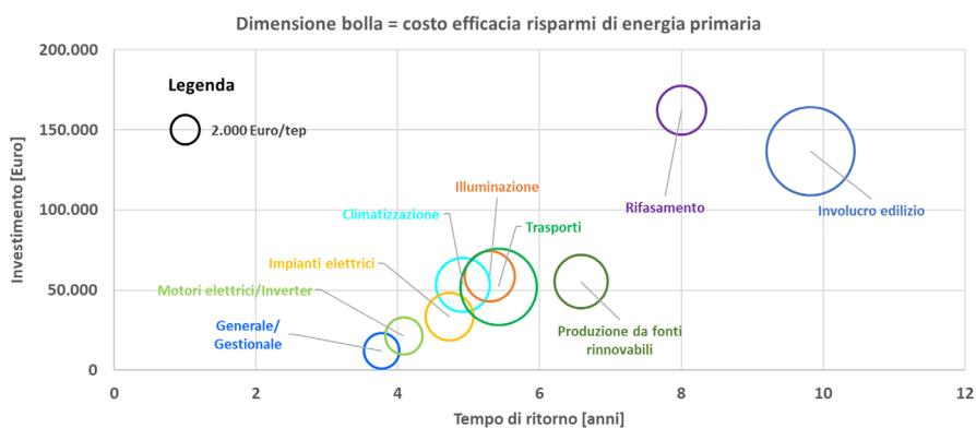
Figura 6.6 – Risparmi potenziali totali di energia primaria: diagramma a bolle con costo efficacia del risparmio energetico, investimento e tempo di ritorno.
